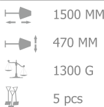
Z18 GRABIE METALOWE 18-ZĘBNE Metal rake 18-teeth
